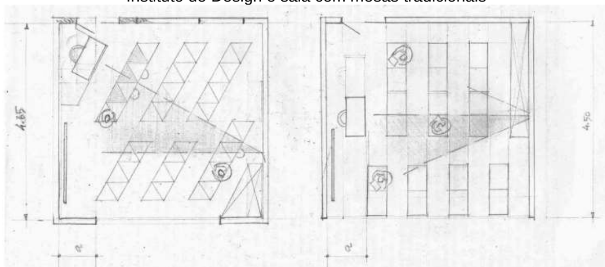
Figura 8 - Projetos comparativos entre sala quadrada equipada com mesas do Instituto de Design e sala com mesas tradicionais
