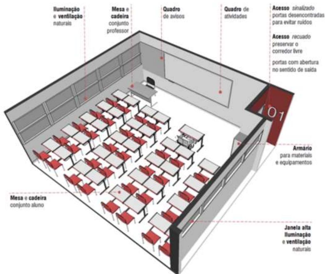
Figura 10 - Layout tradicional sugerido para salas de ensino fundamental
